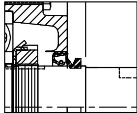
PU LIP SEAL DETAIL
