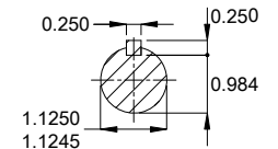
DE Shaft End
