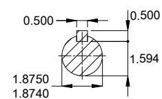
DE Shaft End
