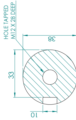
SECTION A-A SCALE 1 : 1
